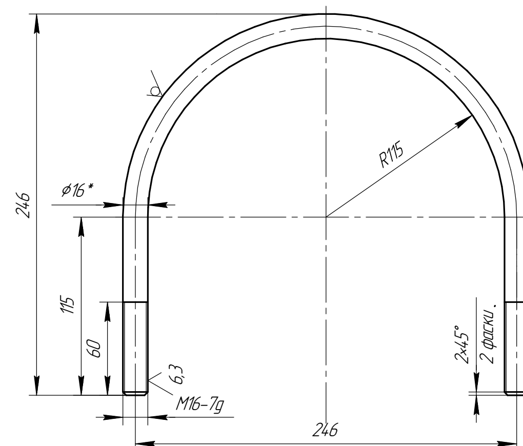
Дет. поз. 5
