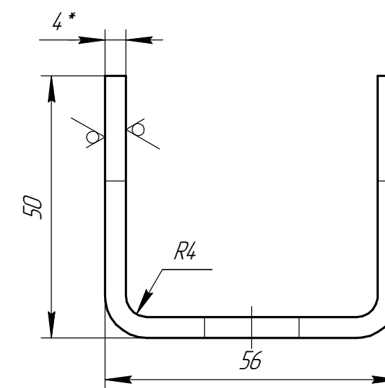
Дет. поз. 3 (1:1)
