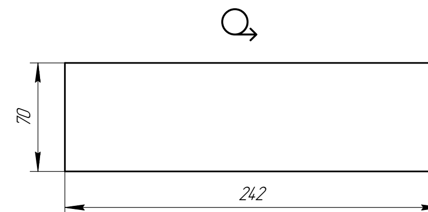
Дет. поз. 4 (1:2)
